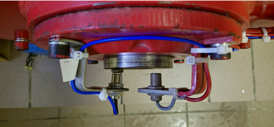
Reparatura ed amplificaziun dad in sensur da mesirar las turas dil generatur, ovra Pardi
